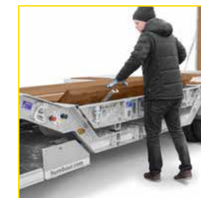
De wielkuipen kunnen indien nodig eenvoudig en flexibel worden vervangen. Voldoende ruimte om de planken op te bergen.
