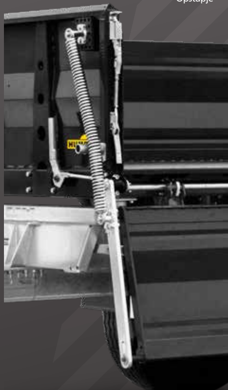
Zijwand opklapbaar met veerontgrendeling
