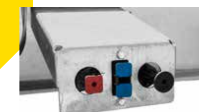
EBS luchtrem met dubbel ontlastventiel, aansluitslangen met rood/gele koppelingkoppen, remsysteem met veerbelaste accumulator
