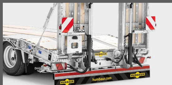
1-sectie hydraulische oprijplaten met hydraulische zijdelings verschuiven
